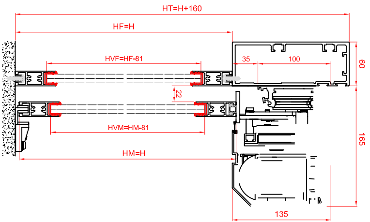
Fijación con Perfil Autoportante Ereka
