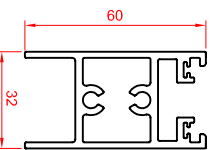
Section Scale: 1/2
