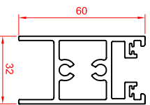
Section Scale: 1/2
